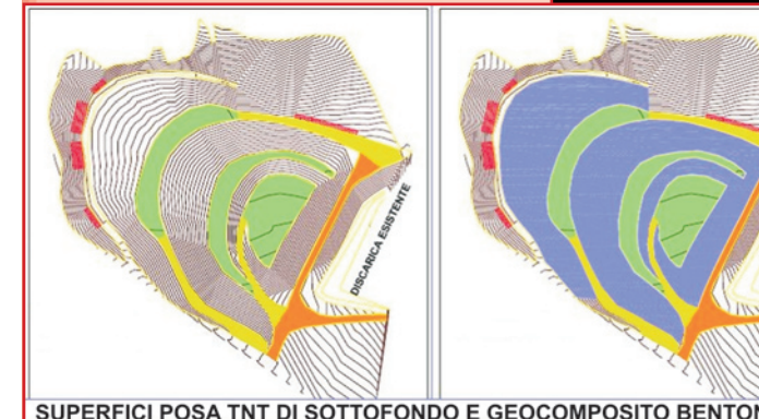
SUPERFICIE POSA TNT DI SOTTOFONDO E GEOCOMPOSITO BENTONITICO
